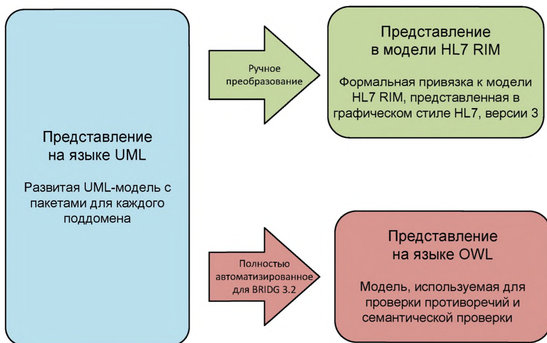
Рисунок 1 — Диаграмма, изображающая использование нескольких представлений в BRIDG
