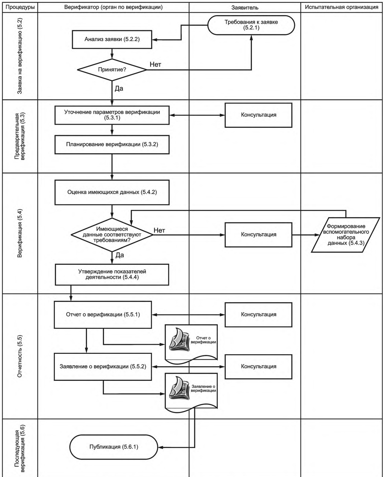
Рисунок В.1 — Блок-схема стандартной ETV-процедуры
