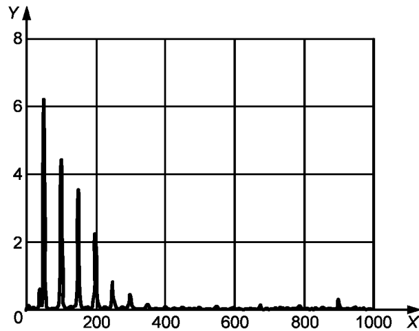
Рисунок В.3 — Ослабление в подшипнике электродвигателя ([2])
