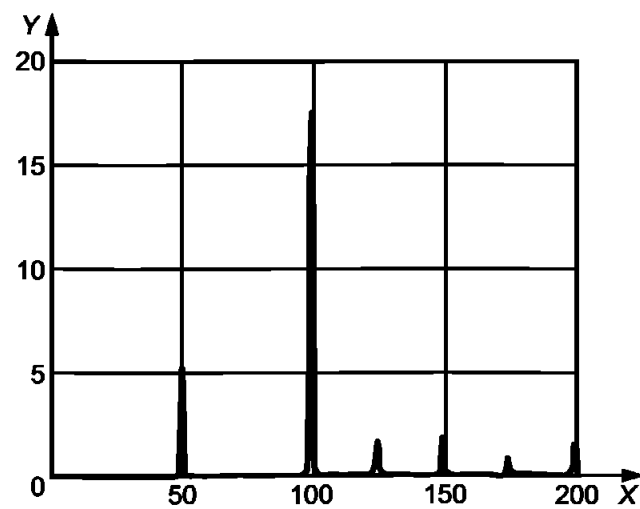
X — частота, Гц; Y — среднее квадратичное значение скорости в вертикальном направлении, мм/с
