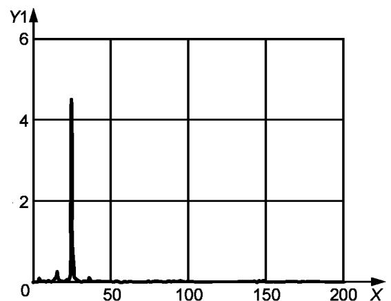
е) Спектр вибрации после внесения изменений
