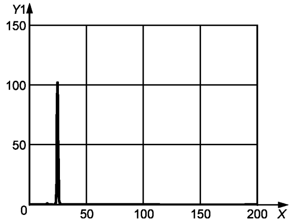
с) Спектр вибрации до внесения изменений
