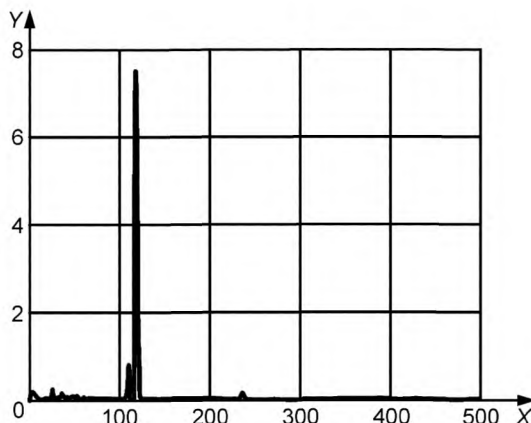
Рисунок В.7 — Увеличенный зазор в подшипнике ([2])
