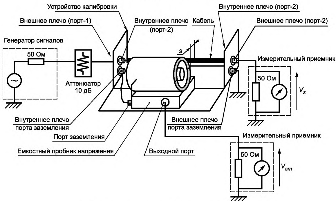
Рисунок G.4 — Модель электростатической связи и её эквивалентная схема
