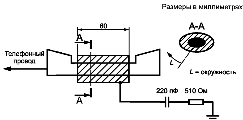
а) Применение эквивалента руки в микротелефонных трубках
