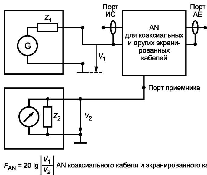
Рисунок F.2 — Установка для испытания коэффициента деления напряжения, дБ, F_{AN} = 20 \lg \left| \frac{V_1}{V_2} \right| АН коаксиально-го кабеля и экранированного кабеля
