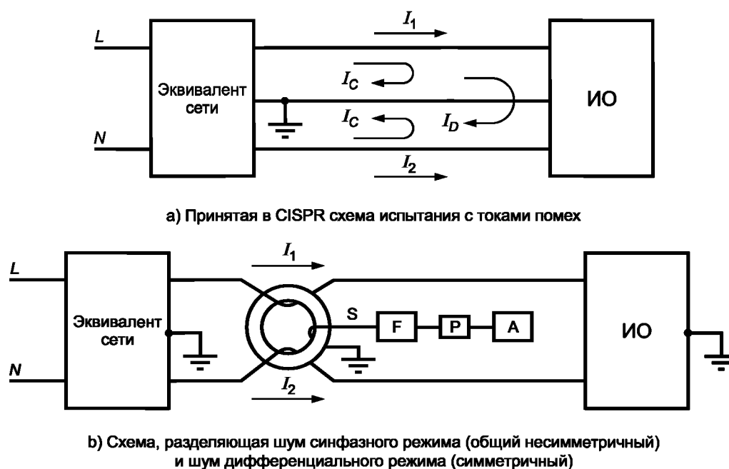
Рисунок В.4 — Испытательная установка для измерения токов с использованием AMN
