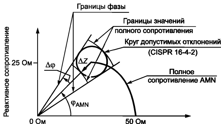
Рисунок I.1 — Определение допустимых отклонений значения и фазы полного сопротивления
