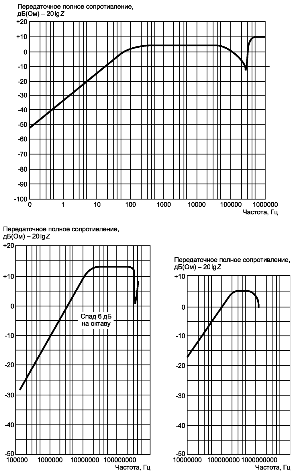
Рисунок В.3 — Передаточное полное сопротивление типовых токосъемников
