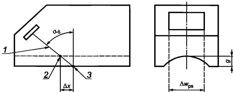
1 — линия, обозначающая смещение точки выхода; 2 — точка выхода луча после профилирования; 3 — точка выхода луча до профилирования
