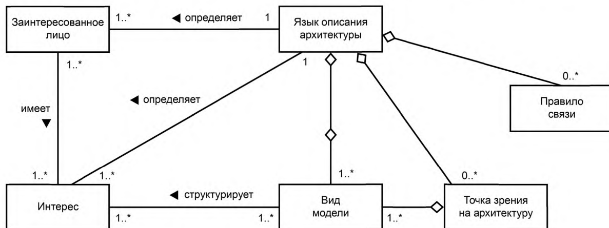
Рисунок 6 — Концептуальная модель языка описания архитектуры
