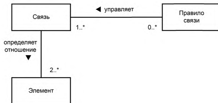
Рисунок 3 — Концептуальная модель элементов и связей описания архитектуры
