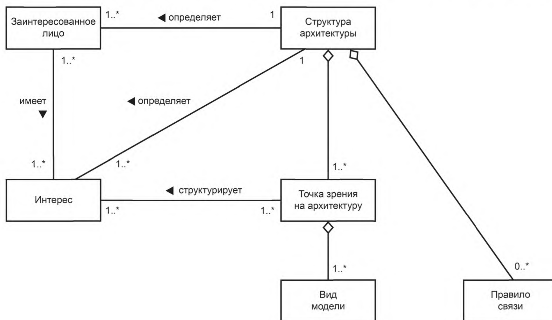
Рисунок 5 — Концептуальная модель структуры архитектуры
