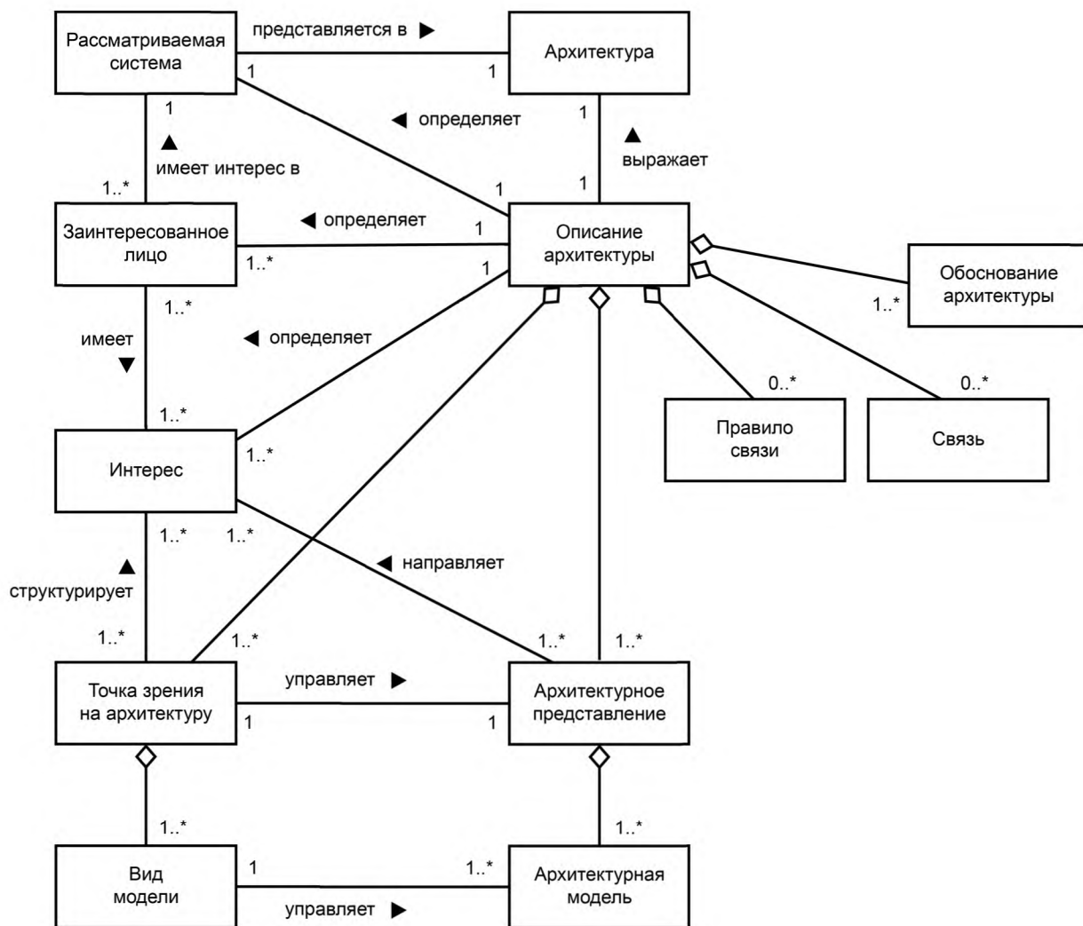
Рисунок 2 — Концептуальная модель описания архитектуры
