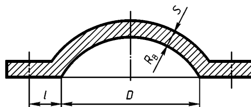
Рис. 8.5.28. Тарельчатое днище
