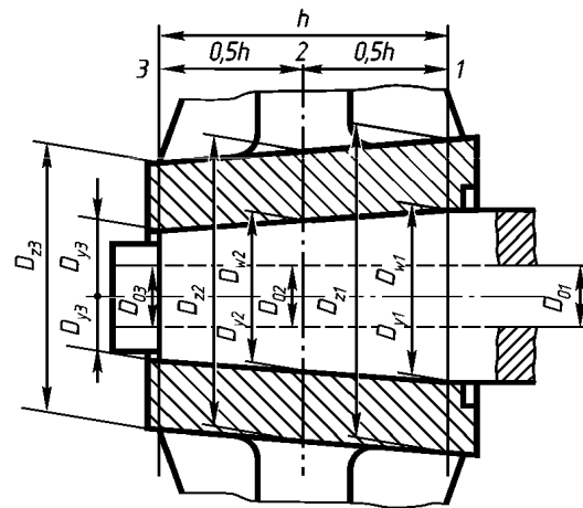
Рис. 3.6.2. К определению осевого перемещения ступицы относительно вала
