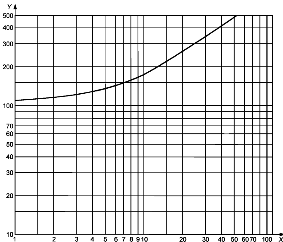
Рисунок 2 — Максимальное напряжение рентгеновской трубки для рентгеновских аппаратов мощностью до 500 кВ как функция от просвечиваемой толщины
