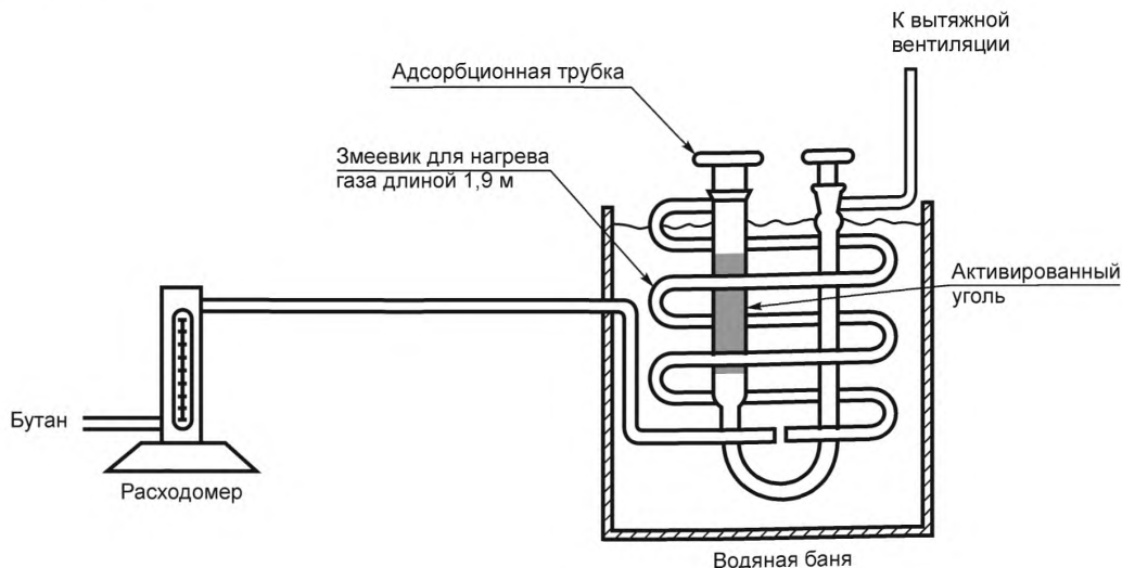
Рисунок 3 — Схема установки для определения активности по бутану
