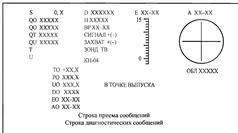
Рисунок 10.8 — Кадр экрана ВКУ в режиме ПОДГОТОВКА
