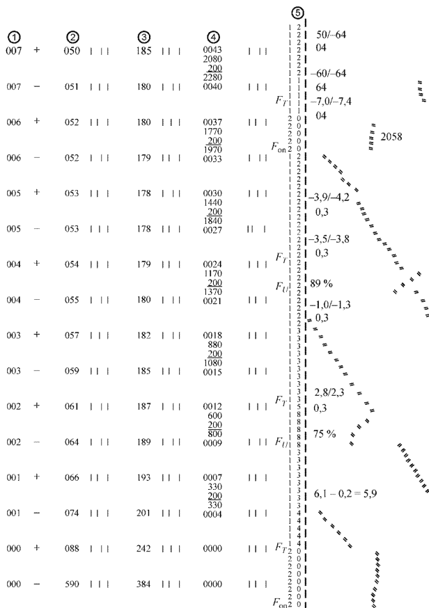
Рисунок 17.1 — Лента регистрации радиолокатора „Метеорит”.
