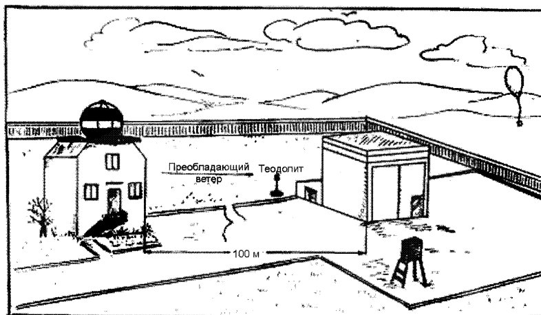
Рисунок 6.1 — Примерный план аэрологической станции
