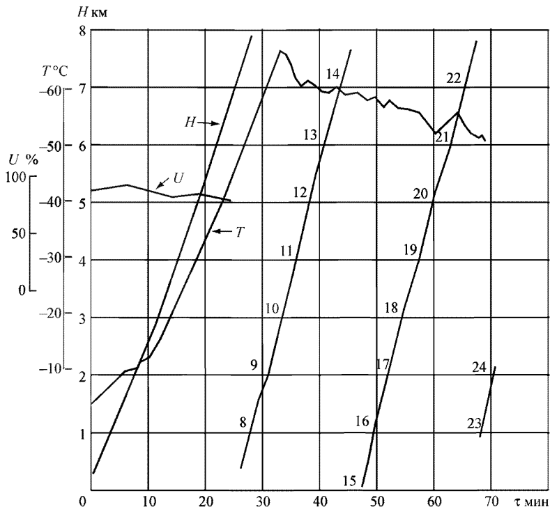
Рисунок 17.2 — График ручной обработки сигналов радиозонда типа МАРЗ
