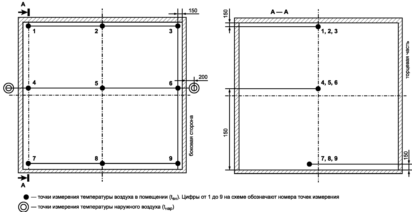
Рисунок А.1 — Схема размещения точек измерения температуры в помещении объемом более 15 м 3 , мм
