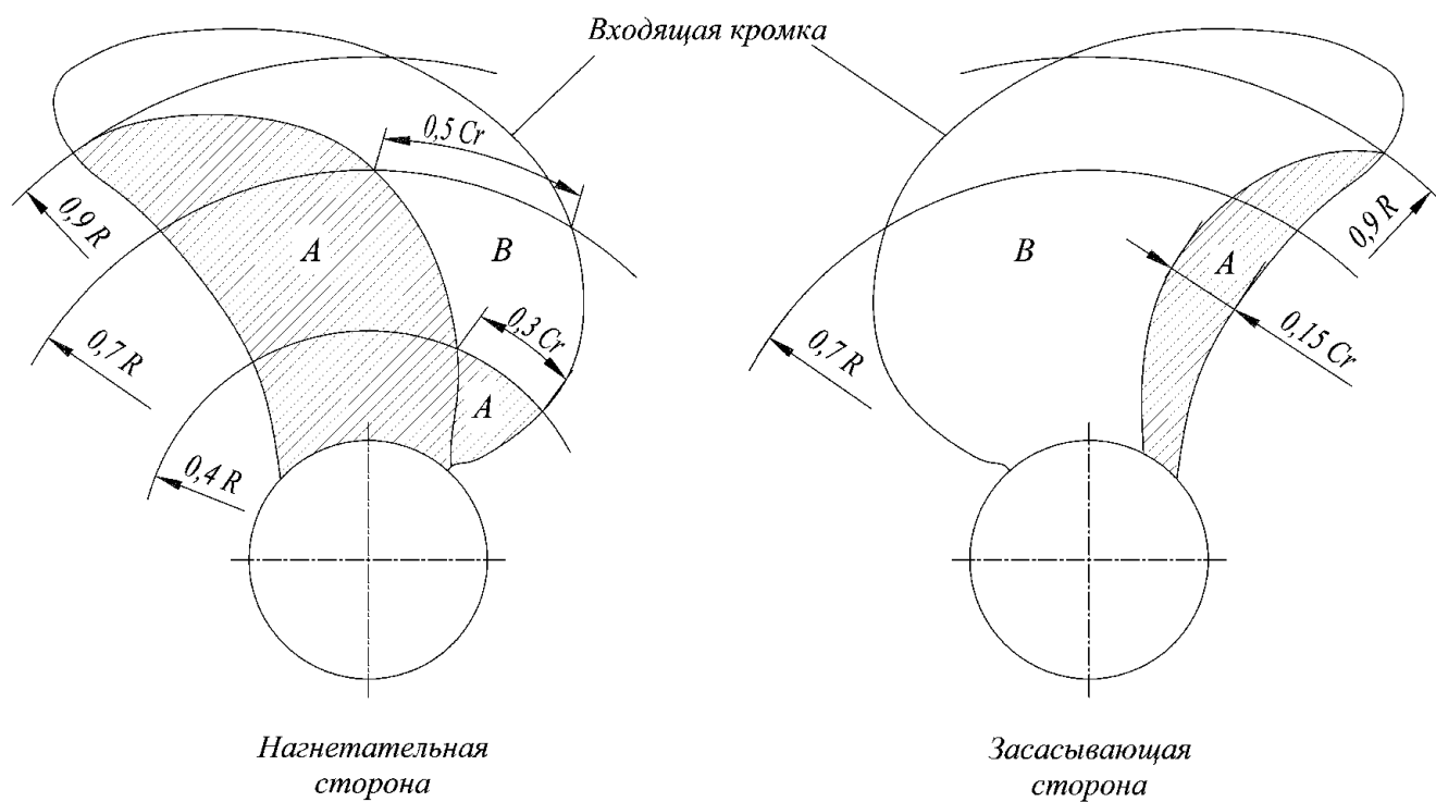
Рис. 4.2.6.3 Зоны контроля в лопастях с откидкой более 25°
