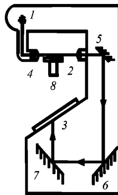
Рис. 2.5.7.2 Прибор, рекомендуемый для определения краевого угла смачивания:
