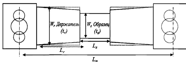
Рис. 3.20.6.2 Схема расположения испытываемого образца, держателя и оснастки
