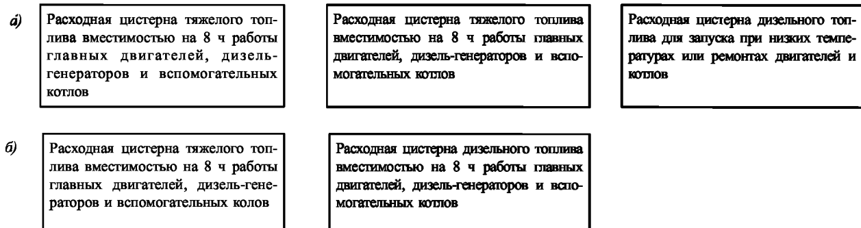
Рис. 13.8.1-1 Расходные цистерны, используемые для подвода топлива к главным и вспомогательным двигателям и вспомогательным котлам, работающим на тяжелом топливе:
