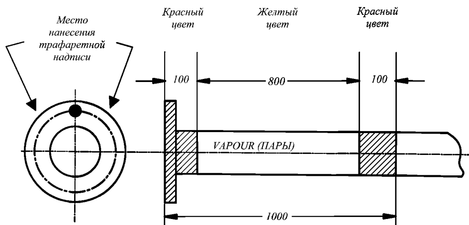
Рис. 6.1.12 Маркировка шланга сдачи паров груза
