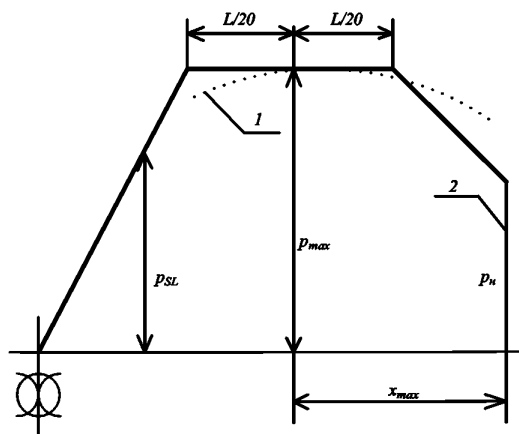
Рис. 2.8.3.2 Схема определения расчетного давления p_{SL} :
