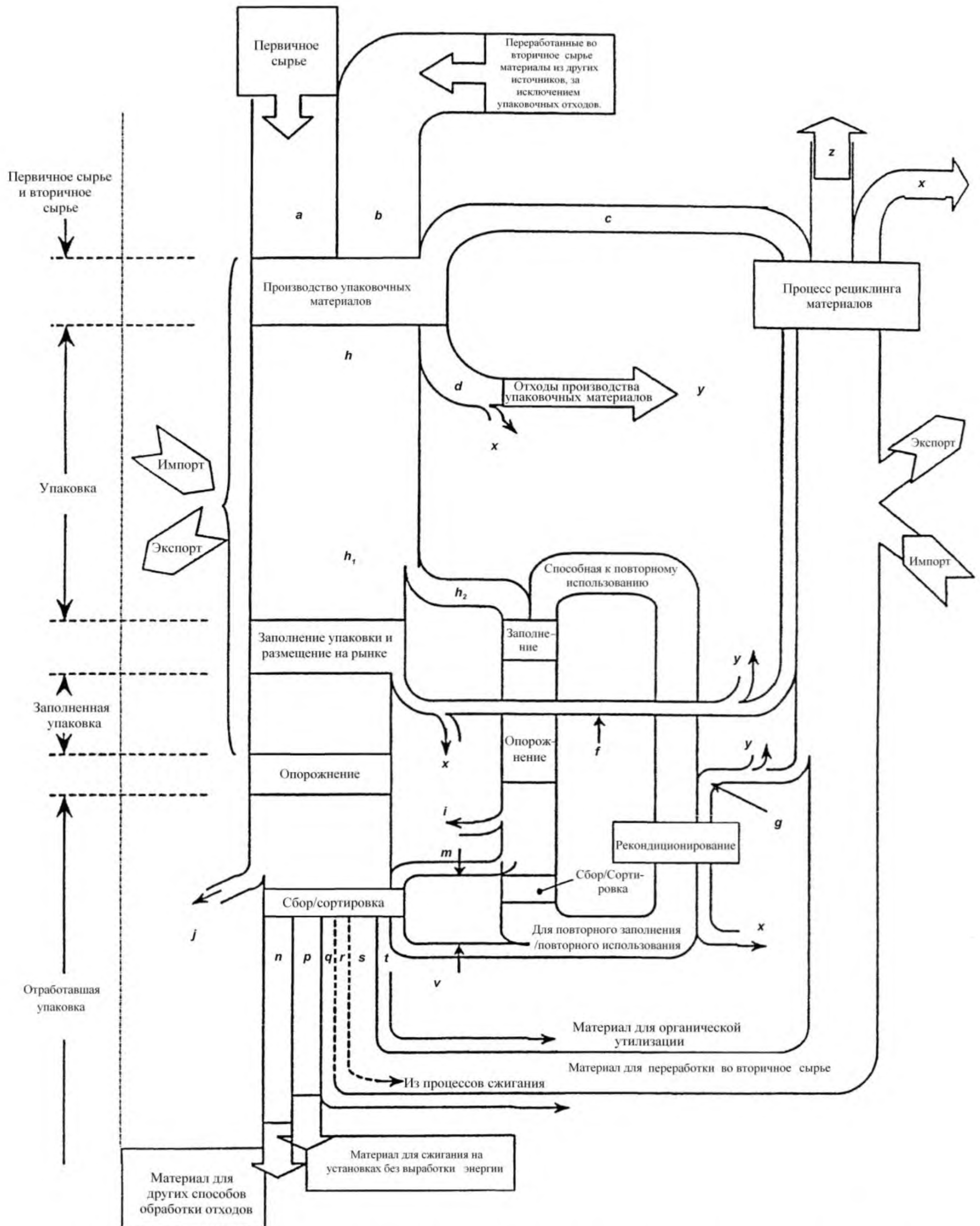
Рисунок А.1 – Поток для переработки упаковки в качестве вторичных материальных ресурсов
