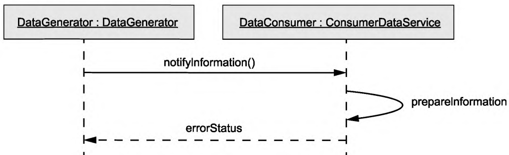
Рисунок 7 — Пример реализации сервиса потребителя
