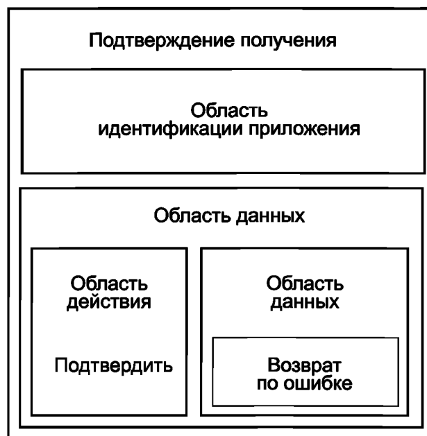
Рисунок А.11 — Сообщение CONFIRM
