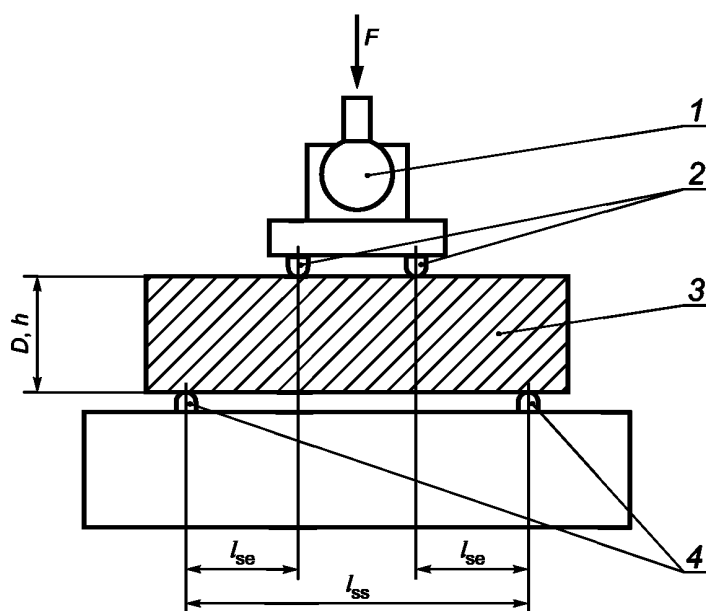
Рисунок 1 — Схема устройства для испытания на изгиб
