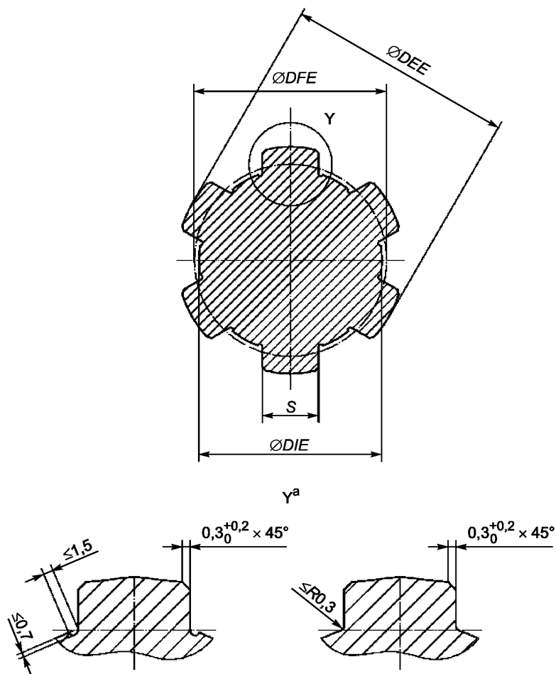
Рисунок 7 — Размеры наружных прямобочных шлицевых зубьев хвостовика ВОМ типа 1
