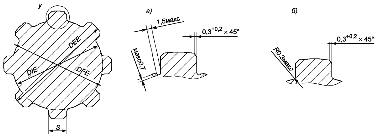
Рисунок 9 — Размеры прямобоочных шлицевых зубьев хвостовика ВОМ типа 1с
