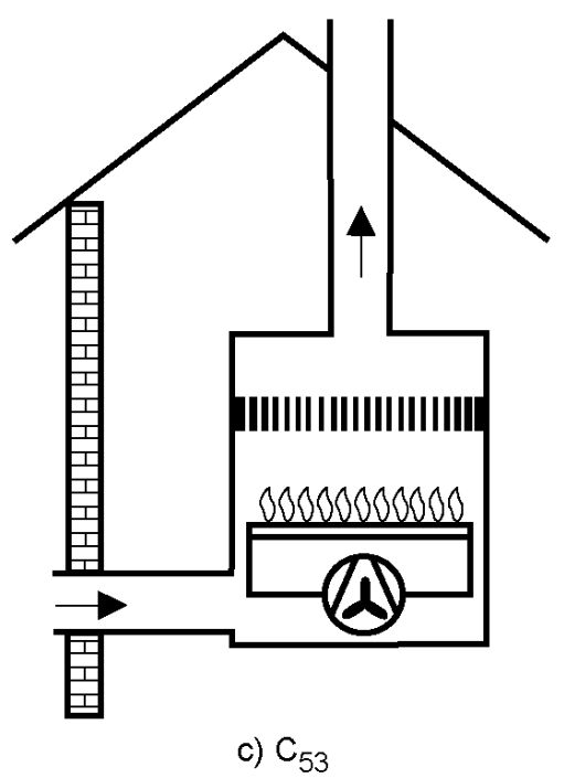
Рисунок D.5 — Тип C 5
