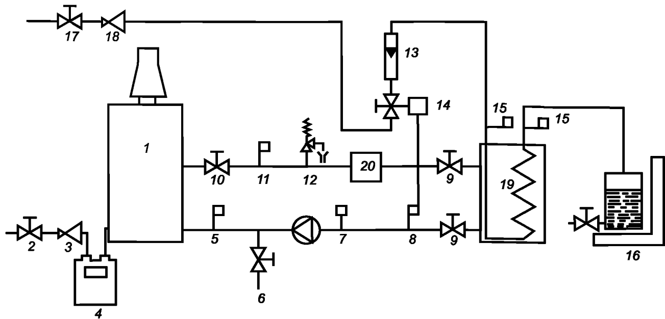
1 – испытуемый котел; 2, 17 – запорный клапан; 3, 18 – регуляторы расхода газа; 4 – счетчик газа; 5, 8, 11, 15 – термометр; 6 – сливной кран; 7 – расширительный бак; 9, 10 – запорный клапан; 12 – предохранительный клапан; 13 – ротаметр; 14 – клапан управления; 16 – весы; 19 – теплообменник; 20 – тепловой компенсатор
