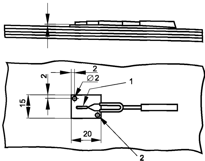
1 – термопара, припаянная к медной пластине; 2 – отверстия для крепления медной пластины
