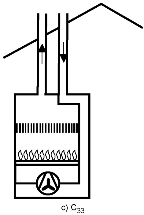
Рисунок D.3 — Тип C 3
