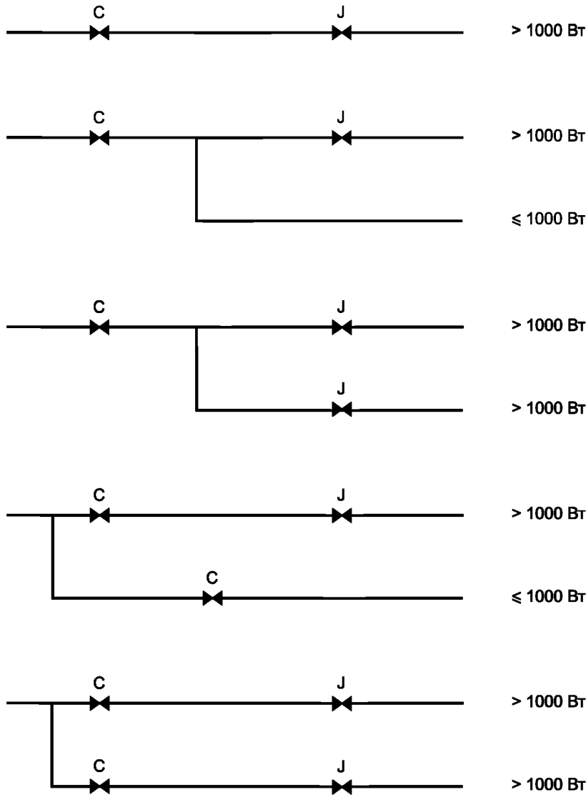
Рисунок Н.1 — Подводимая тепловая мощность до 150 кВт
