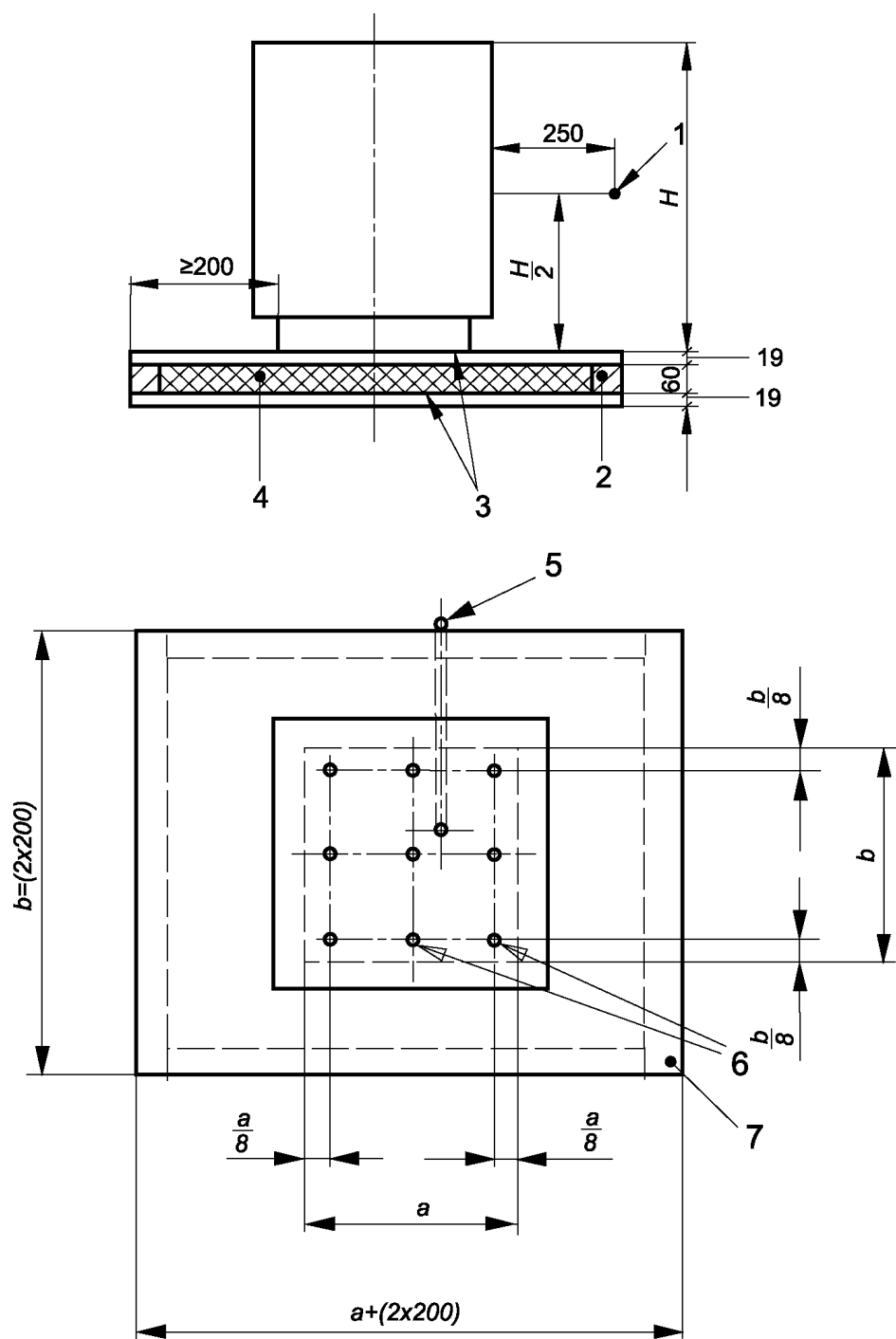
1 – точка измерения температуры воздуха; 2 – рама из четырехгранного бруса; 3 – сосновая доска с пазом; 4 – стекловолокно; 5 – тонкостенная труба для измерительного кабеля; 6 – точки измерений температуры; 7 – испытательная панель для измерения температуры пола под котлом
