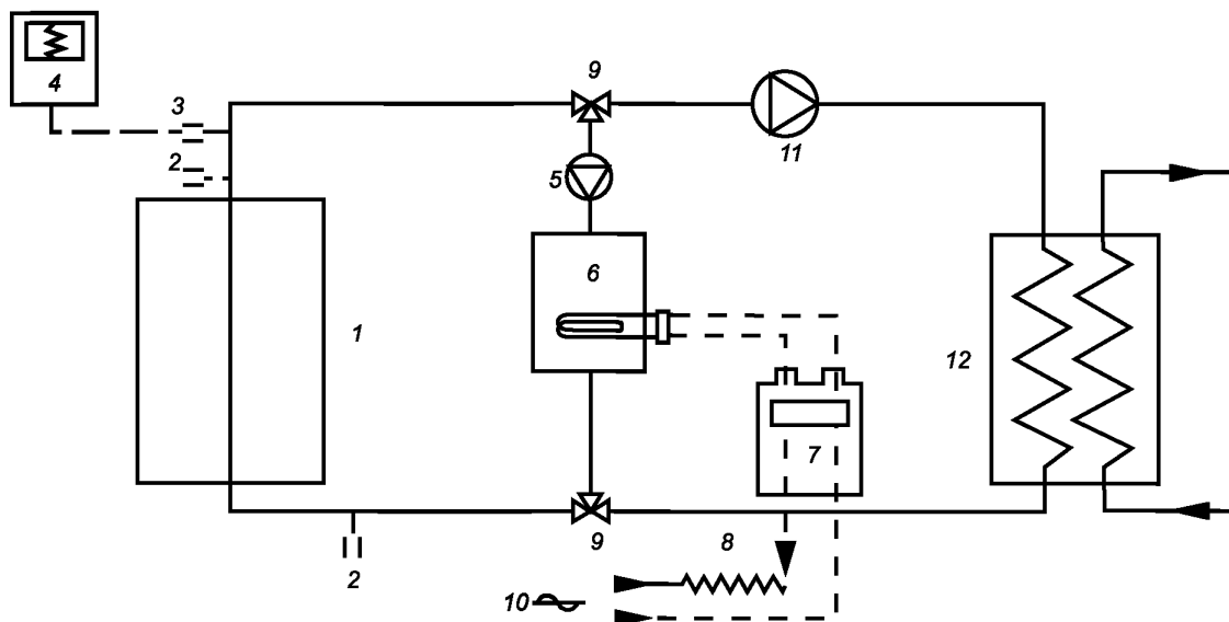
1 – испытуемый котел; 2 – датчик температуры; 3 – низкоинерционный термоземет; 4 – записывающее устройство; 5 – насос (обеспечивает перепад температур между обоими термодатчиками в пределах 2 °С – 4 °С от максимальной испытательной температуры); 6 – электрический водонагреватель; 7 – электросчетчик; 8 – регулятор напряжения; 9 – клапан на 1/4 поворота; 10 – электропитание; 11 – вспомогательный насос (при необходимости); 12 – теплообменник
