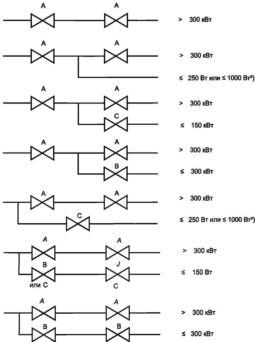
Рисунок Н.6 — Котлы без постоянно или периодически горящей запальной горелки, без системы контроля герметичности клапанов и без предварительной продувки
