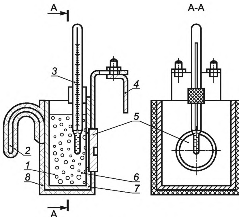
Рисунок 5 — Схема прибора для контроля точки росы
