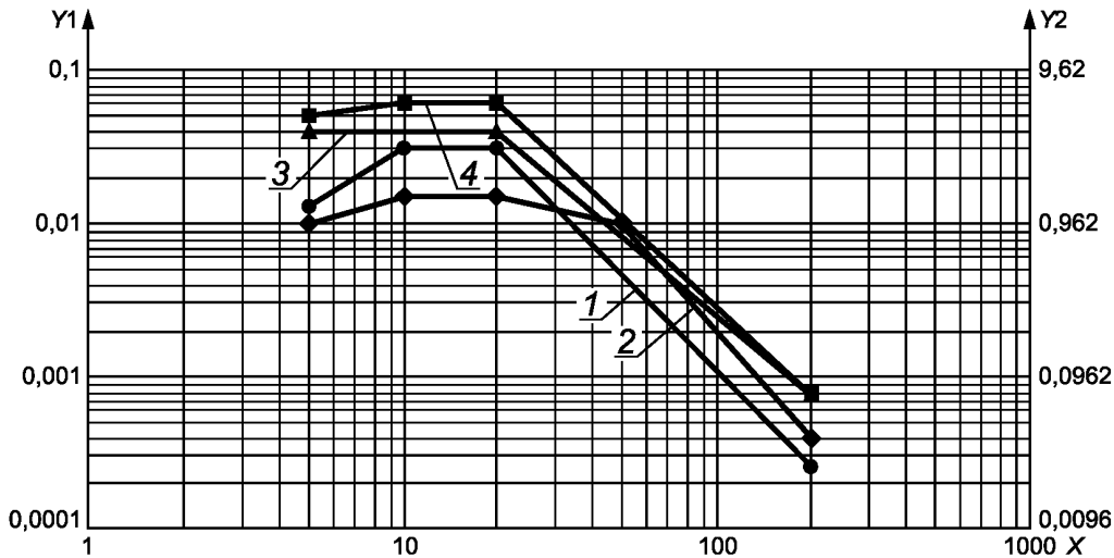
X — частота, Гц; Y1 — спектральная плотность мощности, g 2 /Гц; Y2 — спектральная плотность мощности, (м/с 2 ) 2 /Гц; 1 — СПМ_горизонтальная_продольная_X; 2 — СПМ_горизонтальная_поперечная_Y; 3 — СПМ_горизонтальная_поперечная_Y; 4 — СПМ_вертикальная_Z
