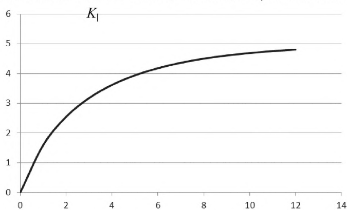
Рисунок А.2 – Зависимость K_I , дБ, от h , дБ
