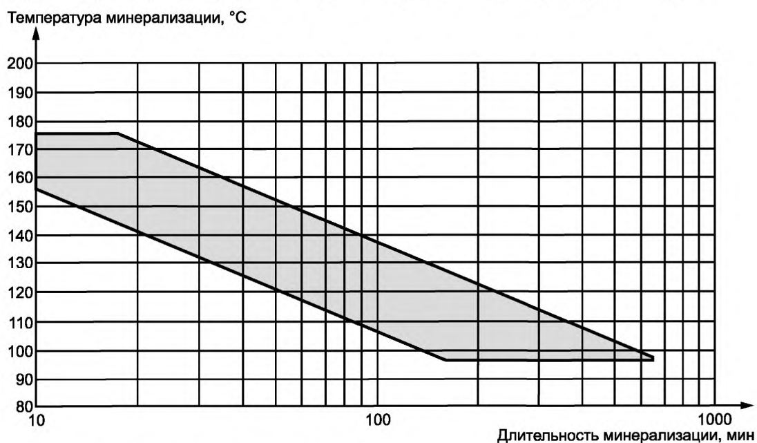
Рисунок 1 — Диапазон допускаемых значений температуры и длительности минерализации
