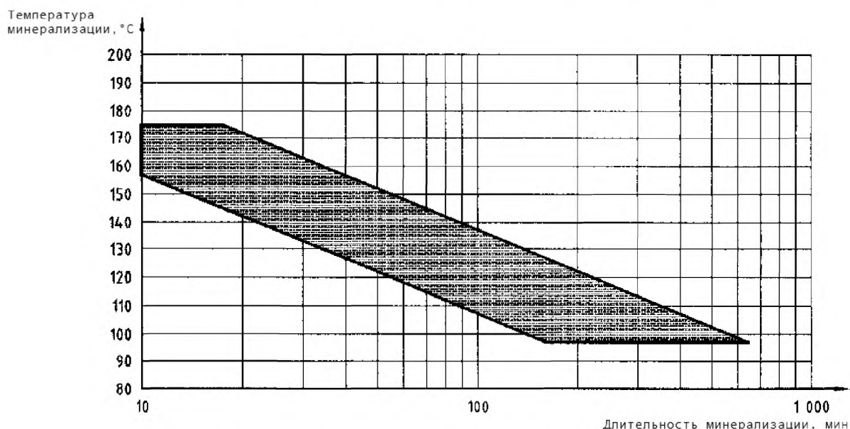
Рисунок 1 — Диапазон допускаемых значений температуры и длительности минерализации
