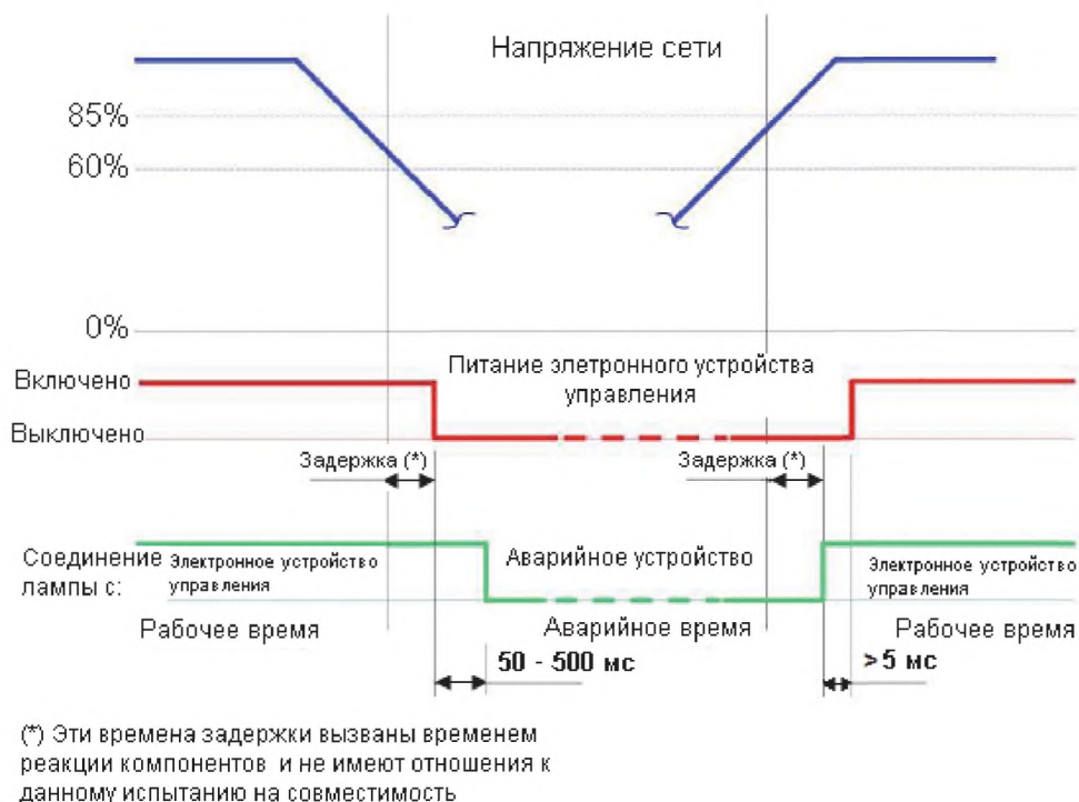
Рисунок L.1 – Временная диаграмма операции переключения
