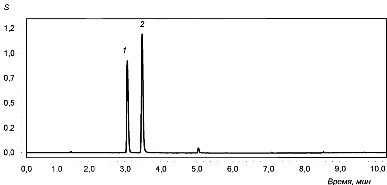
Рисунок В.1 – Хроматограмма градуировочного раствора, содержащего 250 \text{ млн}^{-1} метанола с добавлением 0,01 % по массе внутреннего стандарта 1 – метанол, 2 – внутренний стандарт
