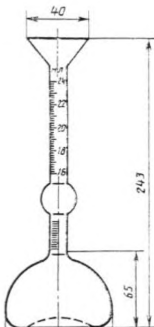
Рисунок 1 – Прибор Ле-Шаталье
