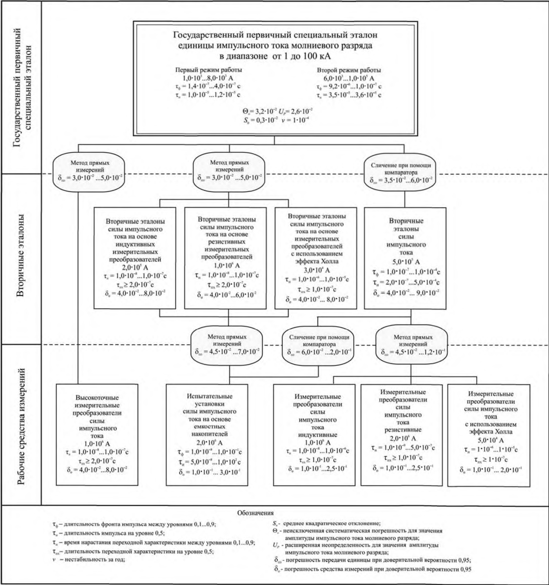
Рисунок А.1 — Государственная поверочная схема для средств измерений силы импульсного тока молниевых разряда в диапазоне от 1 до 100 кА
