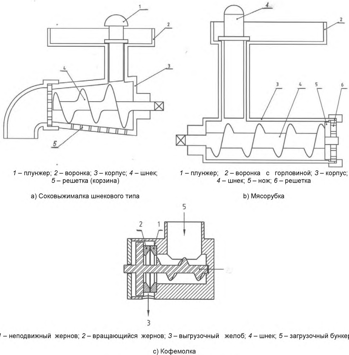
Рисунок 2 – Приспособления шнекового типа
