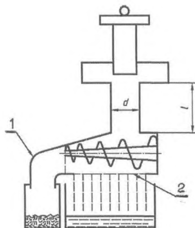
1 – дефлектор; 2 – решетка
