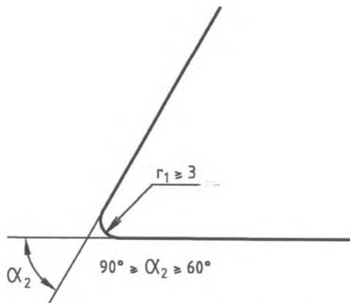
Рисунок А.6 – Зона разбрызгивания (распыления)
