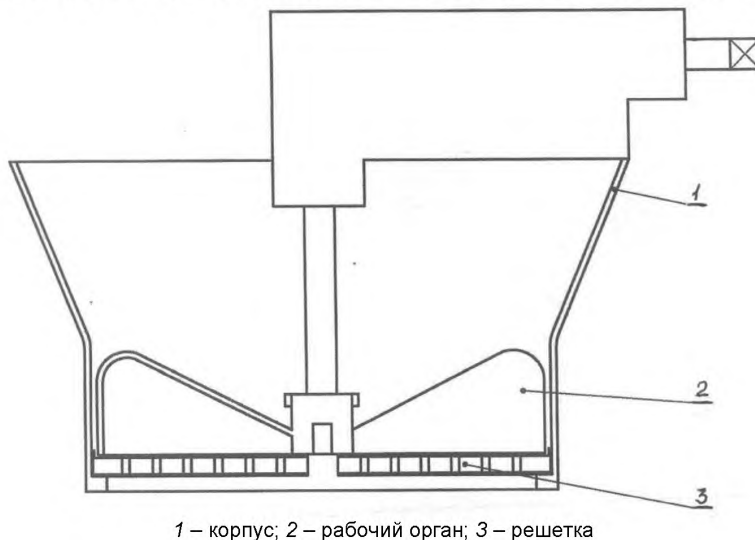
Рисунок 5 – Приспособление для растирания картофеля
