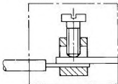
д) винтовой зажим с непрямым давлением
