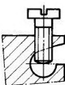
б) винтовой зажим с непосредственным давлением
