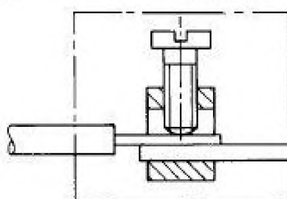
е) винтовой зажим с непосредственным давлением
