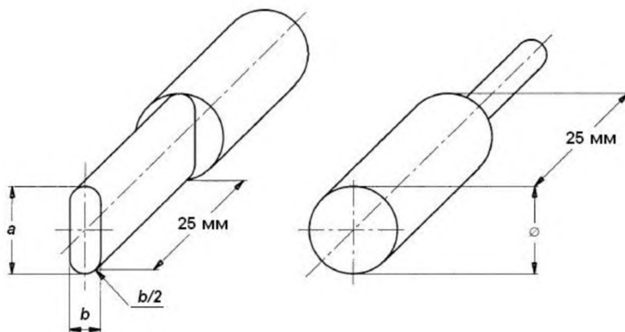
Рисунок АА.1 — Шаблоны для проверки зажимов
