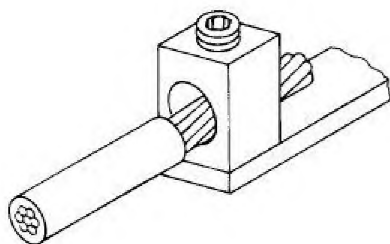
ф) винтовые зажимы с непосредственным давлением
