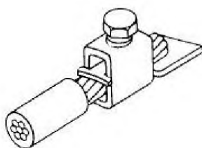
г) винтовой зажим с прижимной пластиной (с непрямым давлением)
