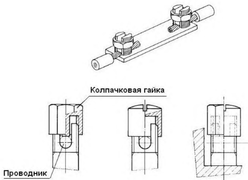
Рисунок 104 — Примеры колпачковых зажимов
