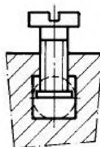
с) с прижимной пластиной
