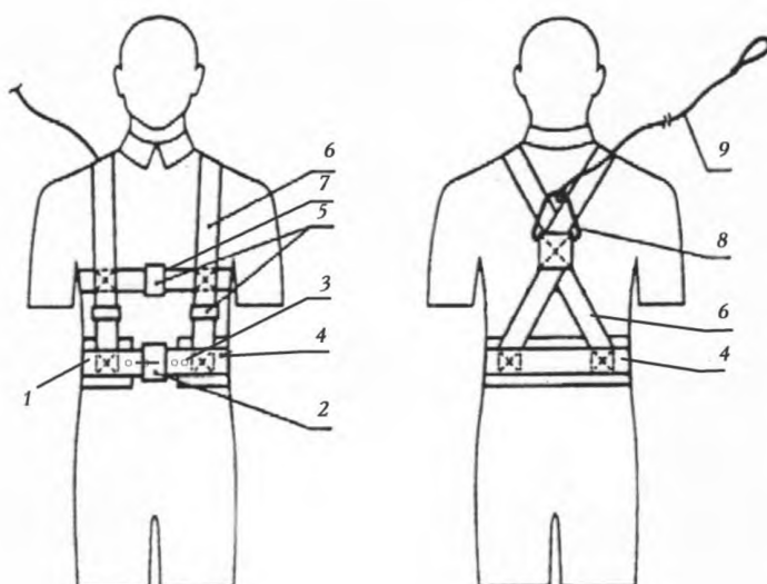
Рисунок 3 – Лямочный пояс, тип В (Ва)
