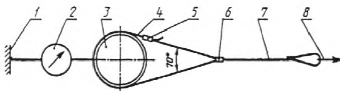
1 – жесткая опора; 2 – измеритель усилия; 3 – цилиндр диаметром 300 мм; 4 – пояс; 5 – пряжка пояса; 6 – боковое кольцо пояса; 7 – строп; 8 – растягивающее усилие
