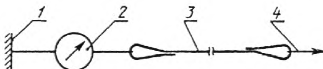
1 – жесткая опора; 2 – измеритель усилия; 3 – строп или другой элемент пояса; 4 – растягивающее усилие
