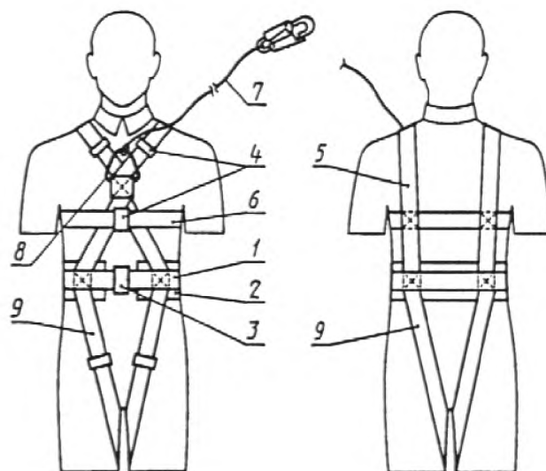
Рисунок 5 – Лямочный пояс, тип Д (Да)
