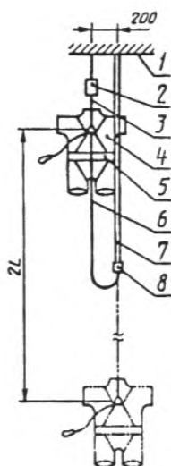
1 — жесткая опора; 2 — сбрасыватель; 3 — соединительное устройство; 4 — манекен; 5 — лямочный пояс; 6 — стропы; 7 — штанга; 8 — серьга штанги;
