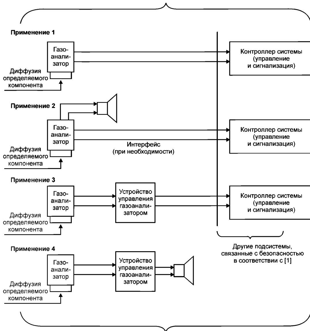
Рисунок А.1 — Газоаналитические подсистемы, связанные с безопасностью
