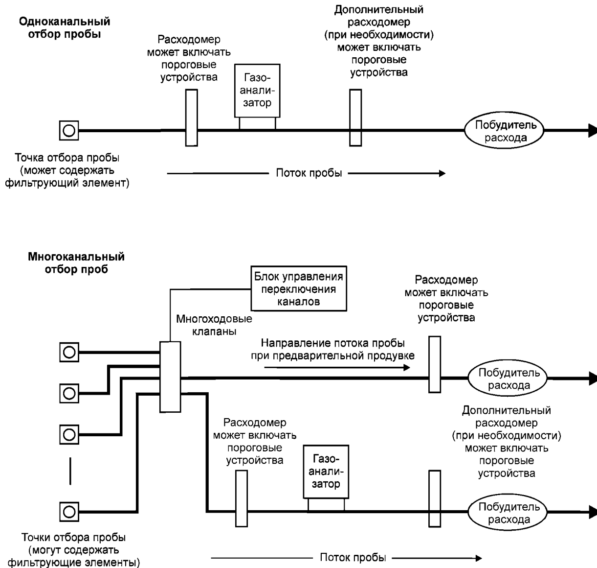
Рисунок А.2 — Типичные конфигурации пробоотборных линий
