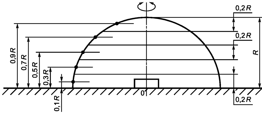
Рисунок А.2 — Соосные круговые траектории микрофона
