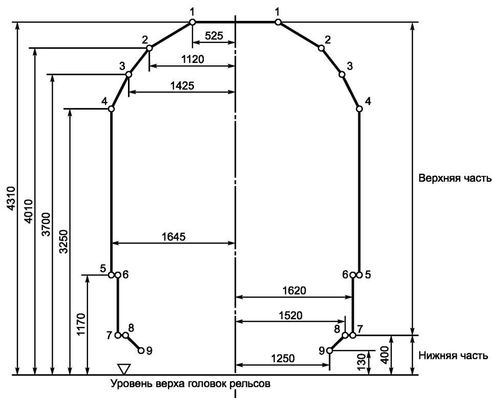
Рисунок 14 — Кинематический габарит 03-ВМ к
