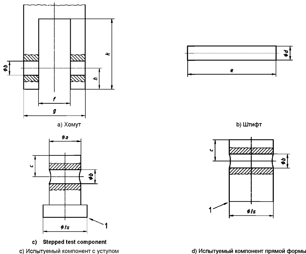
Рисунок 2 – Размеры нагрузочного блока и испытуемых компонентов
