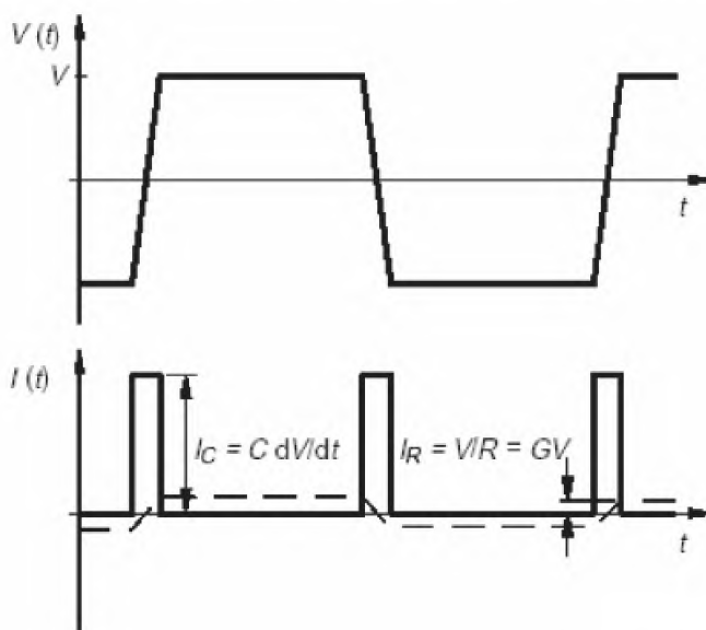
Рисунок 1 – Принцип метода с использованием прямоугольного сигнала
