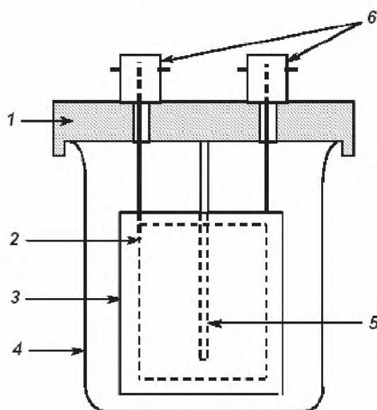
1 – крышка; 2 – внутренний электрод; 3 – внешний электрод; 4 – сосуд из нержавеющей стали; 5 – карман для измерения температуры; 6 – разъемы BNC для электрических соединений
