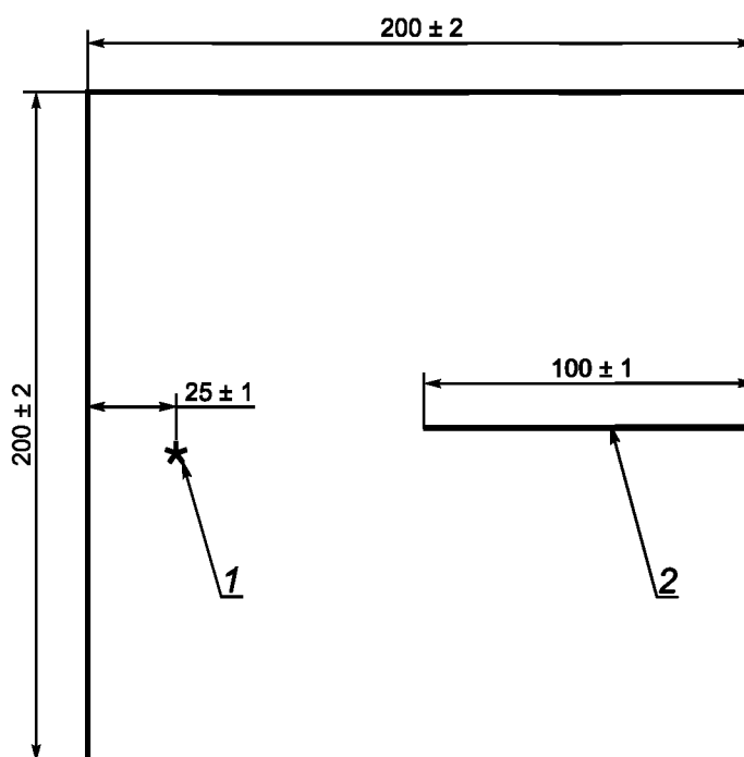
Рисунок D.1 — Широкие испытываемые образцы в форме брюк
