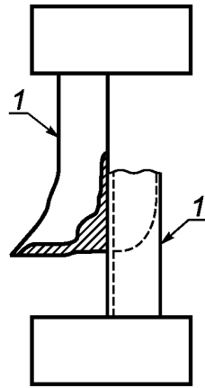
Рисунок D.2 — Зажим испытываемых образцов в зажимных устройствах
