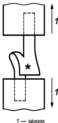
Рисунок 2 — Зажимное устройство
