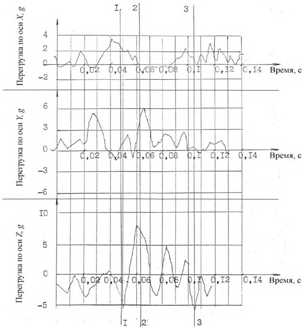
Рисунок 7 — Пример совмещенной диаграммы ускорений (перегрузок) в центре масс автомобиля по осям X, Y и Z
