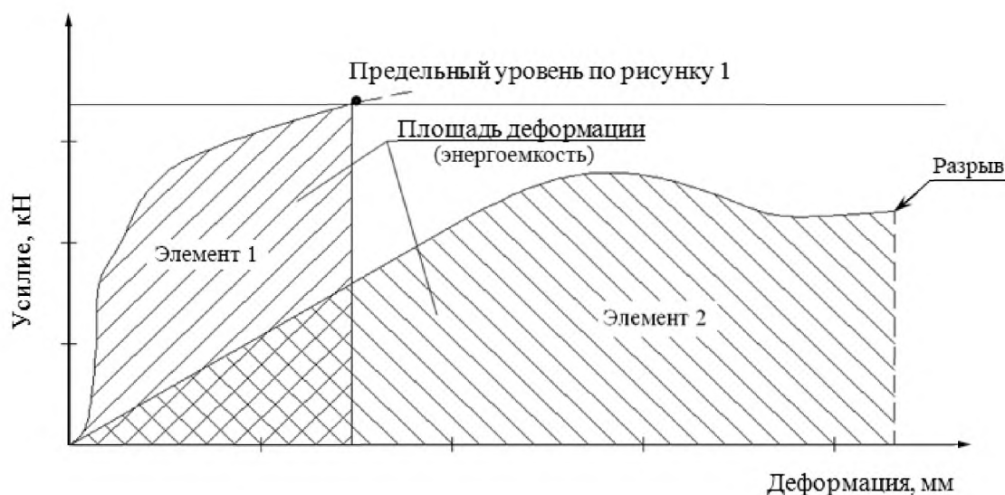
Рисунок 2 — Примеры диаграмм деформации элементов (фрагментов) барьерного ограждения при различных случаях завершения испытаний по 5.3.1
