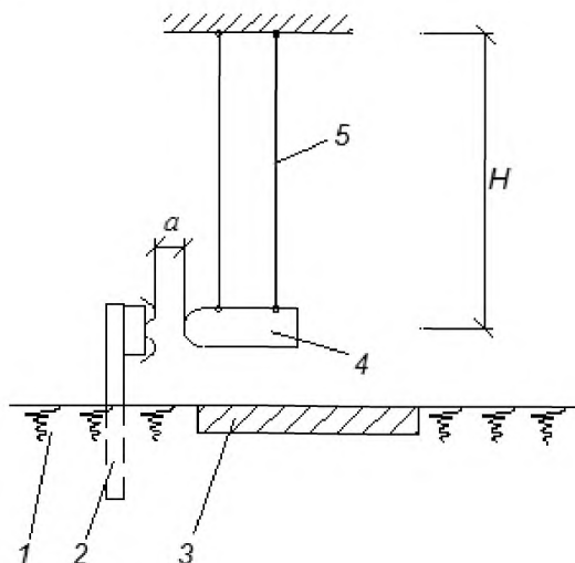
1 — грунтовое основание, 2 — стойка дорожного ограждения, 3 — жесткое основание, 4 — боек, 5 — подвеска, H — высота маятника, a — размер, определяемый по 6.2.2
