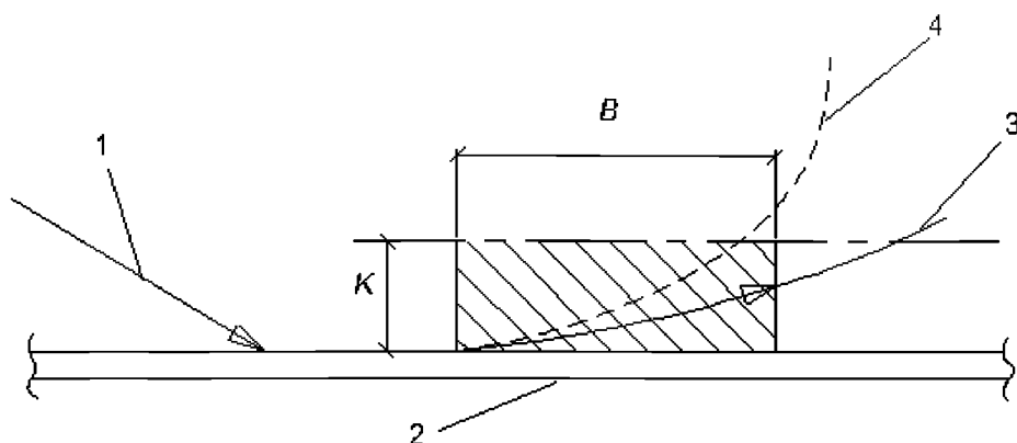
1 — траектория наезда, 2 — ограждение, 3 — траектория выбега, удовлетворяющая требованиям безопасности, 4 — траектория выбега, не удовлетворяющая требованиям безопасности
