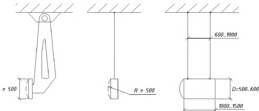
а — жесткая подвеска, б — гибкая одиночная подвеска, в — гибкая сдвоенная подвеска
