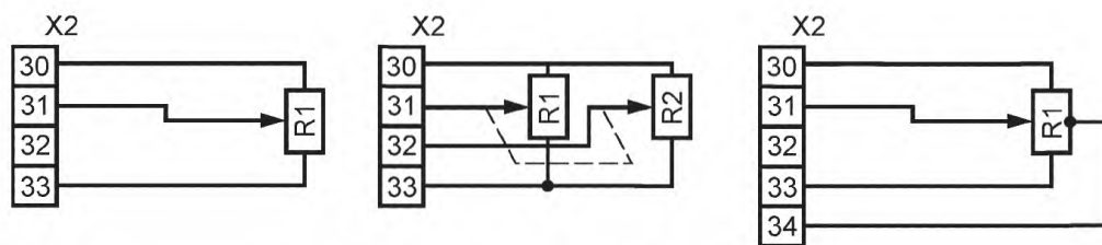
Схема подключения резистивных датчиков
