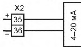
Схема подключения токового датчика
