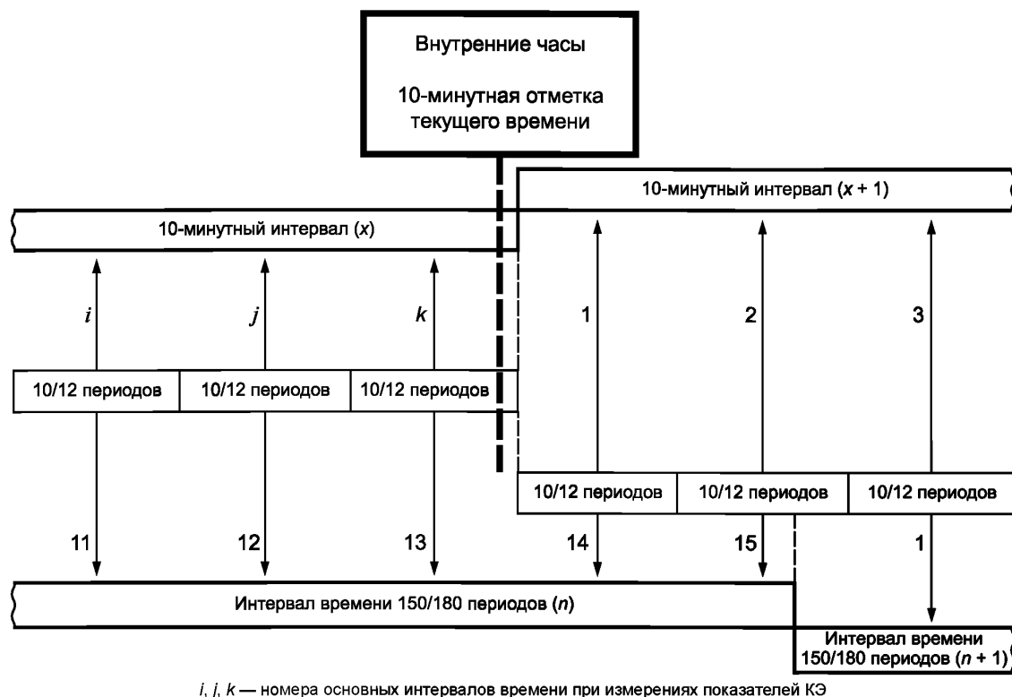
Рисунок 3 — Синхронизация объединенных интервалов для класса S: измерение показателей КЭ, для которых пропуски недопустимы
