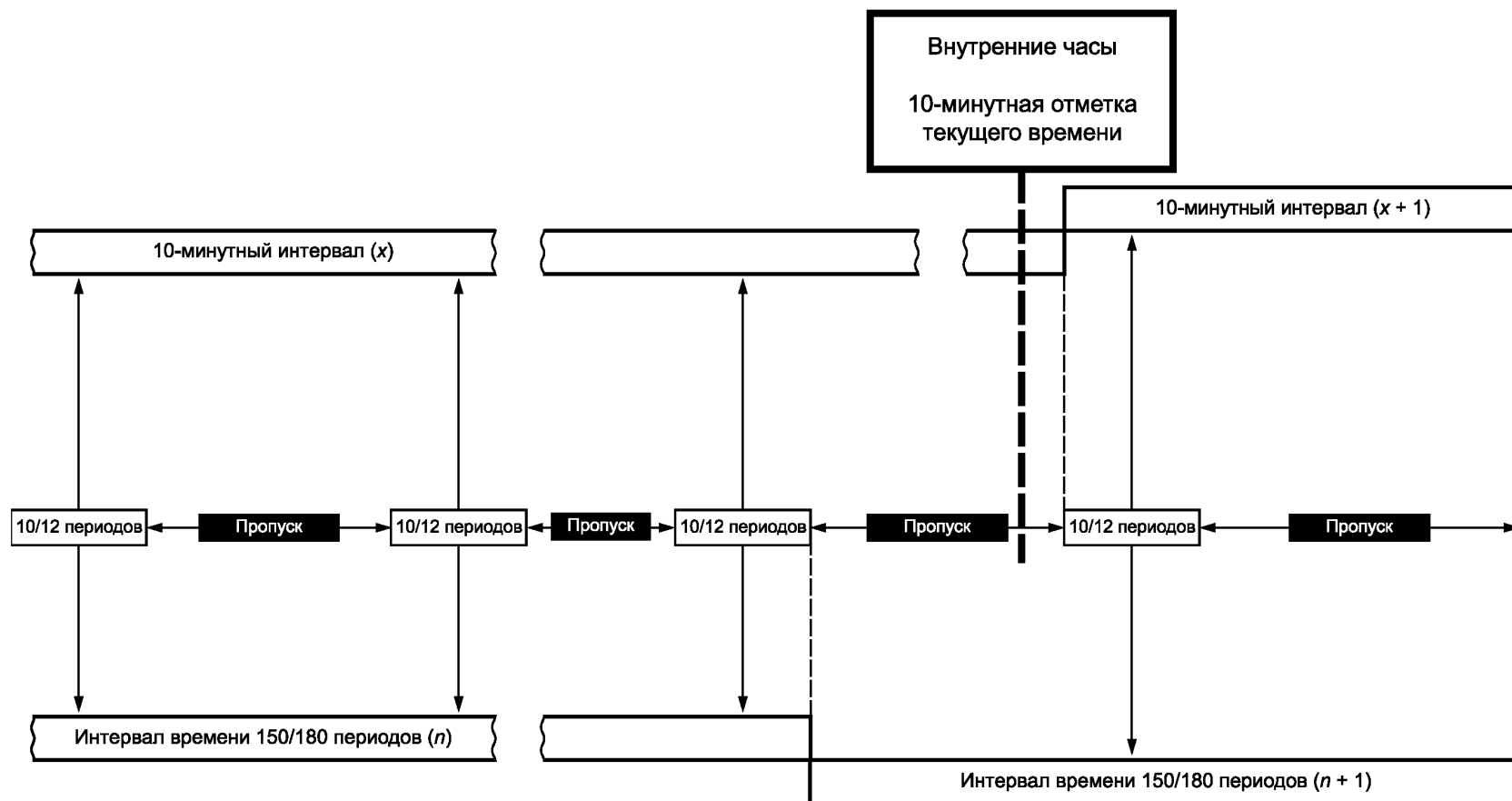
Рисунок 4 — Синхронизация объединенных интервалов для класса S: измерение показателей КЭ, для которых пропуски допускаются
