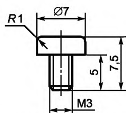
Верхняя часть центрального проводника. Нержавеющая сталь. Приблизительно 2:1
