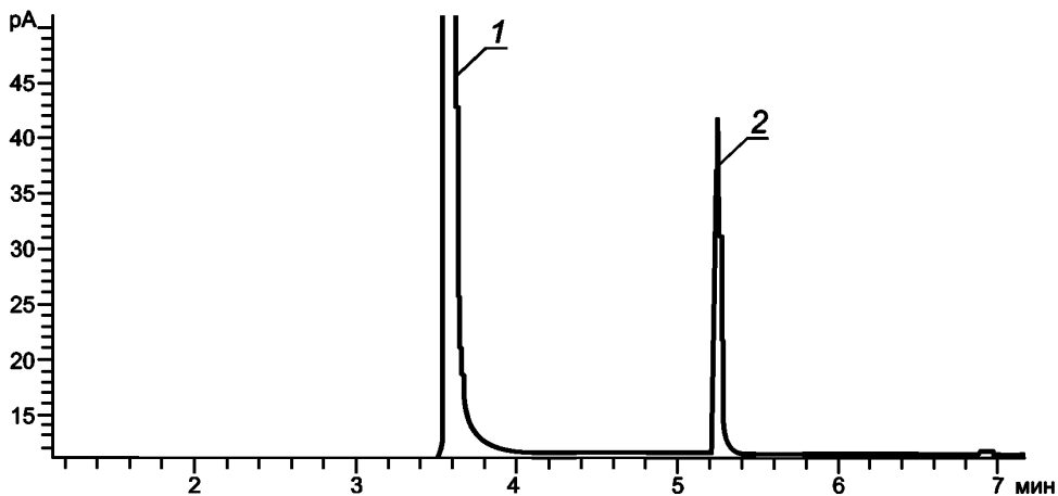
1 — этиловый спирт; 2 — кротоновый альдегид
