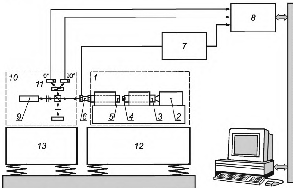
1 — ударный стенд (см. 4.2); 2 — пружинный элемент; 3 — молоток на воздушной опоре; 4 — прокладка; 5 — наковальня (например, из стали диаметром 30 мм и длиной 200 мм) на воздушной опоре; 6 — акселерометр; 7 — усилитель; 8 — цифровой регистратор формы сигнала (см. 4.8); 9 — лазер (см. 4.5); 10 — интерферометр (см. 4.6); 11 — фотодетектор (см. 4.6); 12 — первый сейсмический блок (см. 4.4); 13 — второй сейсмический блок (см. 4.4)
