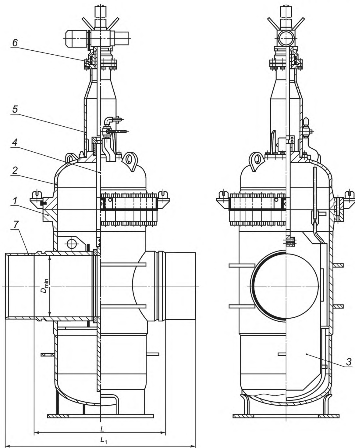
1 — корпус; 2 — крышка; 3 — шибер; 4 — шпindelь; 5 — стойка; 6 — бугельный узел; 7 — приварная катушка
