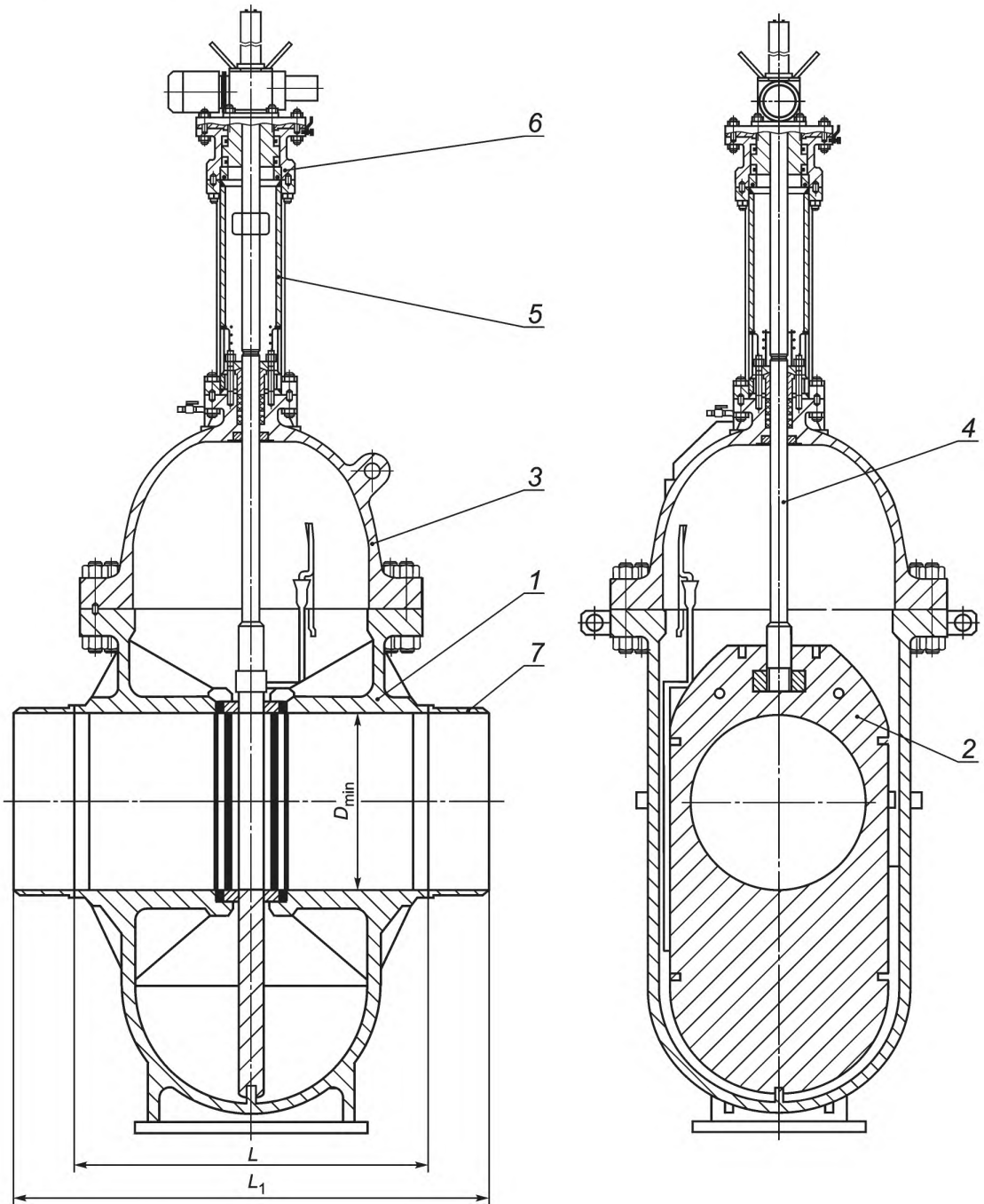
1 — корпус; 2 — шибер; 3 — крышка; 4 — шпindelь; 5 — стойка; 6 — бугельный узел; 7 — приварная катушка
