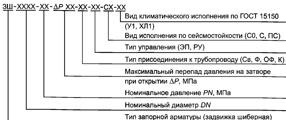
Рисунок 1 — Схема условного обозначения задвижек
