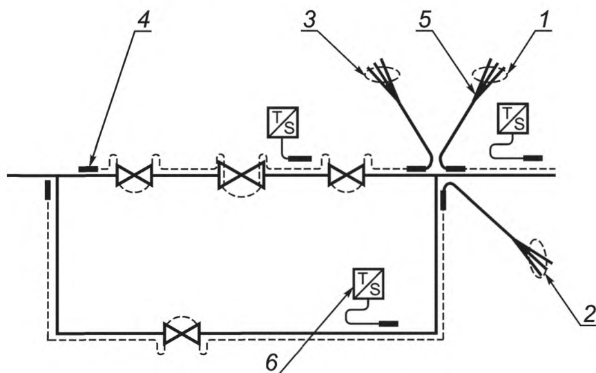
1 — цепь № 1; 2 — цепь № 2; 3 — цепь № 3; 4 — заделка горячего конца; 5 — заделка холодного конца; 6 — температурный датчик
