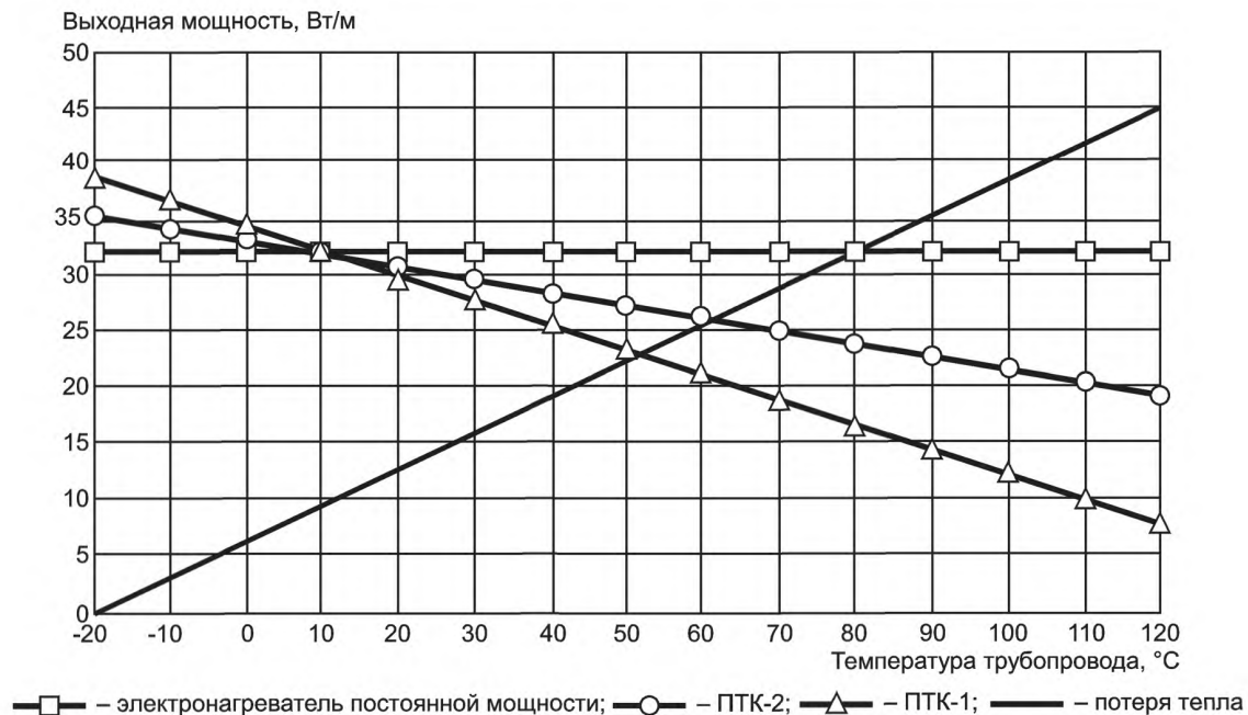
Рисунок 3 — Условия равновесия для поддержания температуры в трубопроводе
