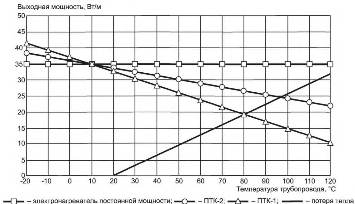
Рисунок 4 — Условия равновесия для оценки верхнего предела
