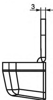
Рисунок Б.18 — Пример запорной планки для накладного замка
