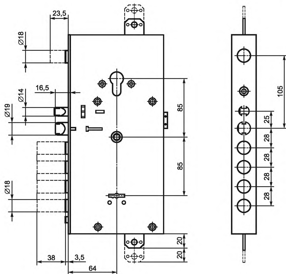
Рисунок Б.7 — Пример комбинированного врезного электромеханического замка
