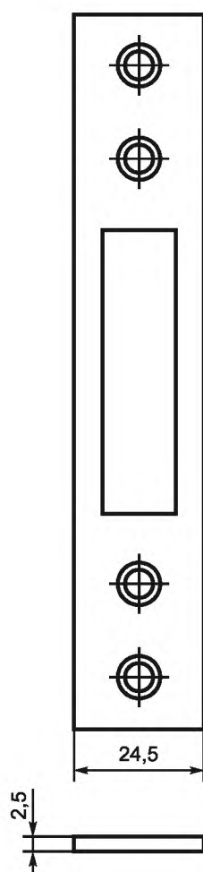
Рисунок Б.14 — Пример простой запорной планки
