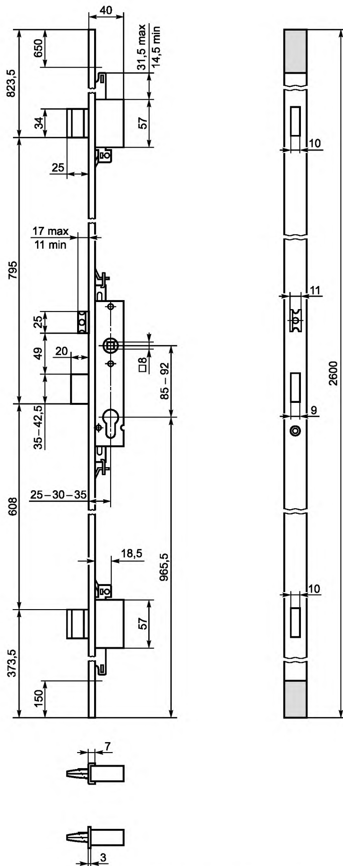
Рисунок Б.22 — Пример многозапорного замка
