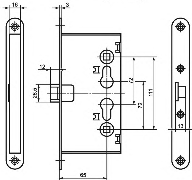
Рисунок Б.12 — Пример замка для противопожарной двери
