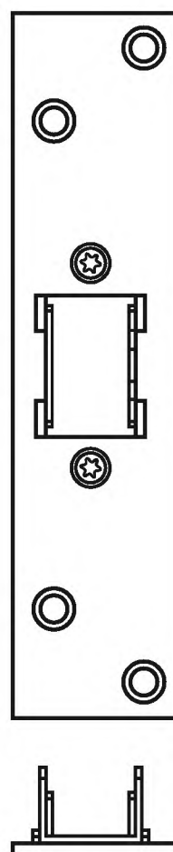
Рисунок Б.15 — Пример запорной планки с усиленной зоной захода засова
