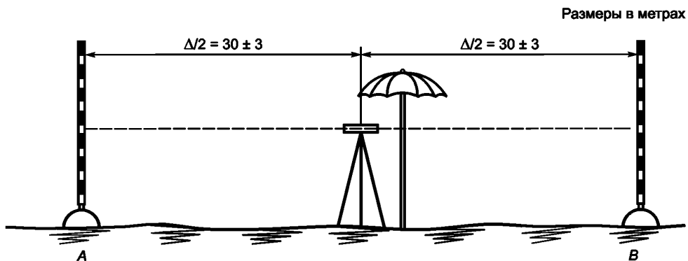
Рисунок 3 — Конфигурация хода для полной методики испытания
