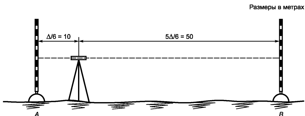
Рисунок 2 — Вторая конфигурация хода для упрощенной методики испытания
