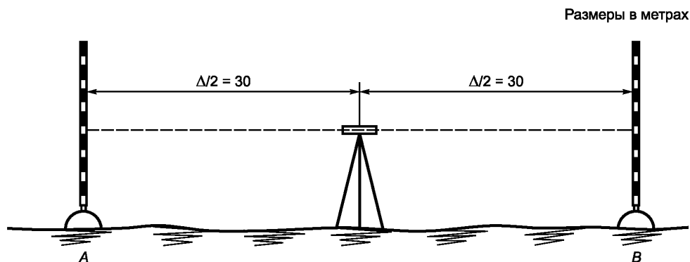
Рисунок 1— Первая конфигурация хода для упрощенной методики испытания
