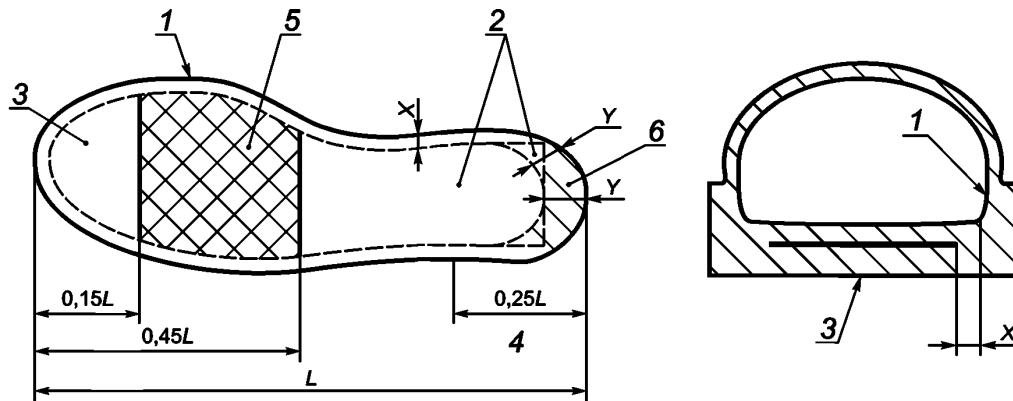
1 — линия шва на отливке; 2 — вариант формы вставки; 3 — антипрокольная прокладка; 4 — область пятки; 5 — заштрихованный участок; 6 — заштрихованный участок 2; L — внутренняя длина нижней части обуви
