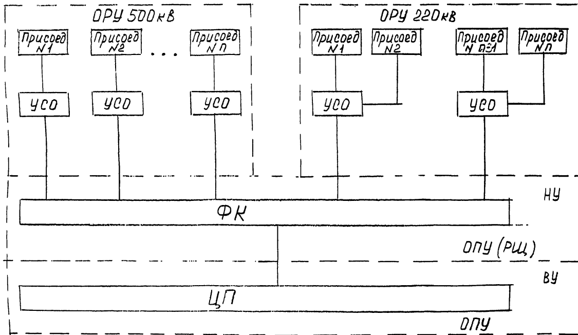
Рис 1. Структура блокировки оперативных переключений в составе АСУ ТП ПС.
