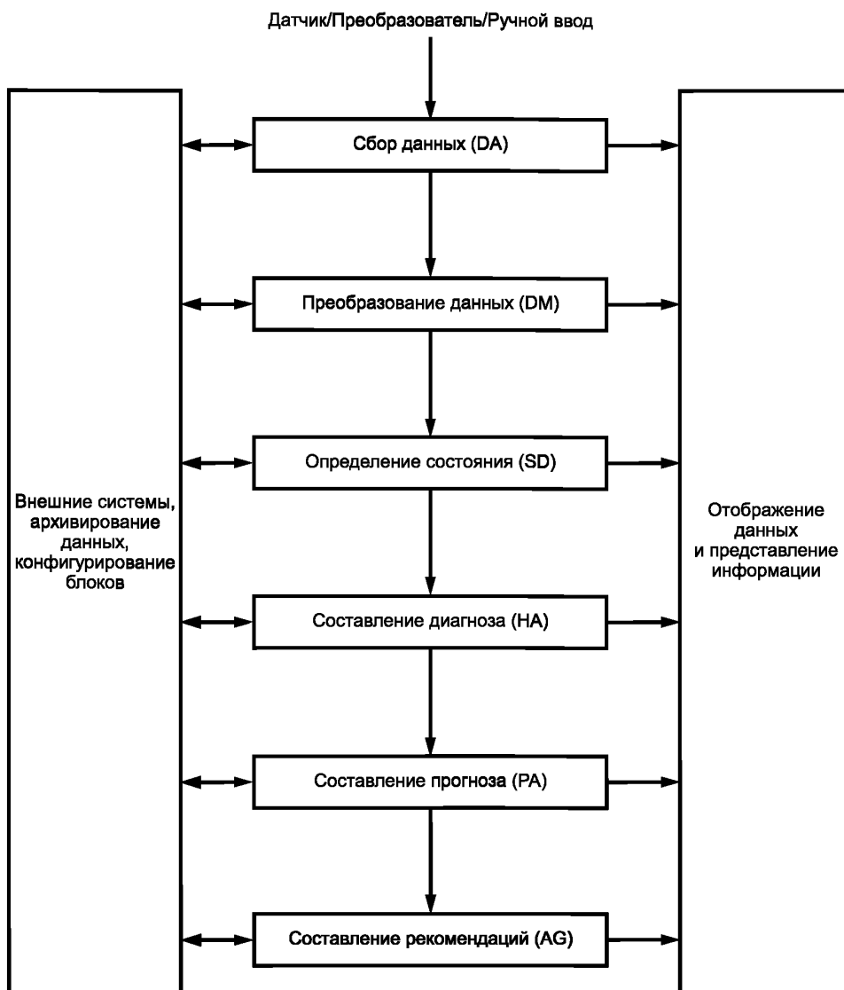
Рисунок 2 — Блок-схема этапов обработки данных
